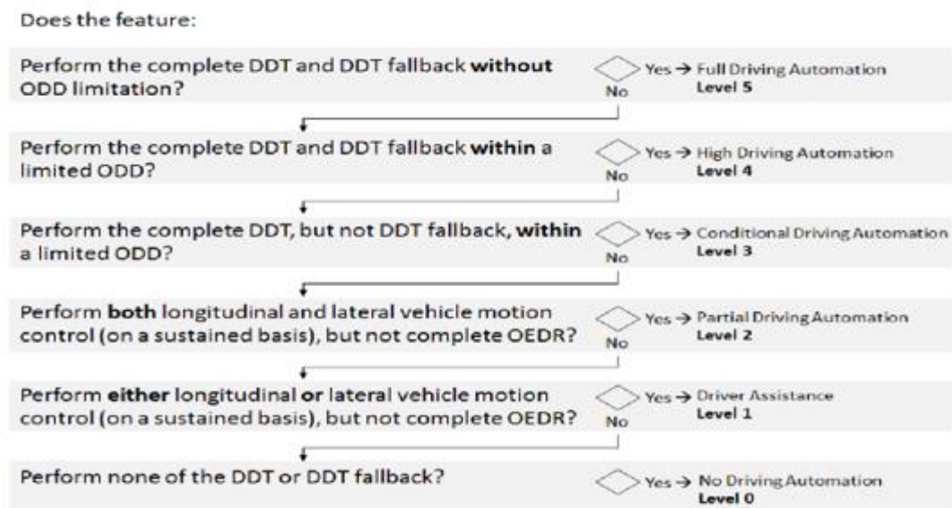
Imagen 2: Diagrama de flujo lógico simplificado para asignar el nivel de automatización de la conducción a una función.
